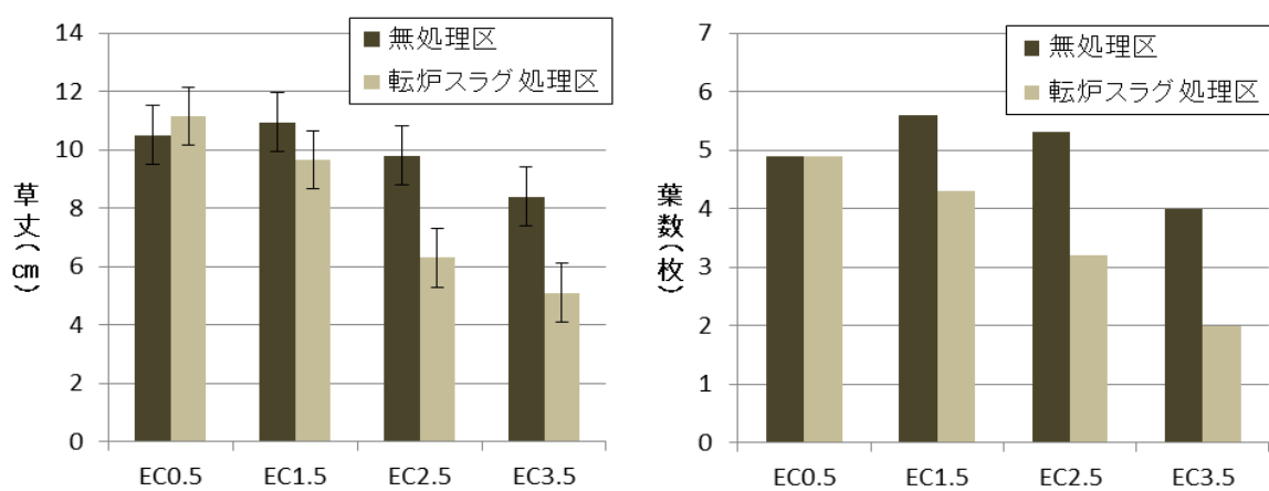
図7 EC別土壌における播種27日後における生育調査結果（ポット試験、左：草丈、右：葉数）
