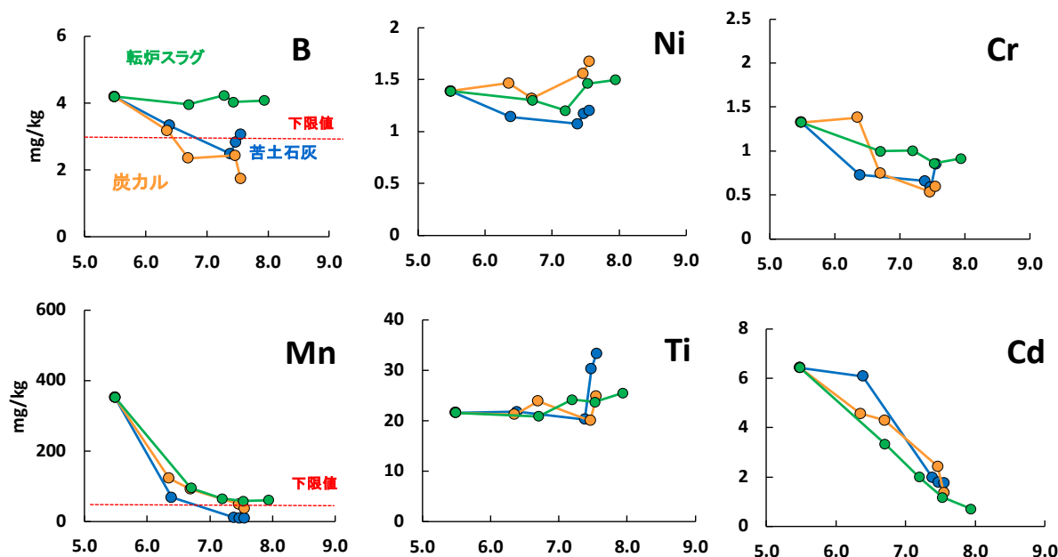
図5 酸性改良資材の違いがソルゴーの微量元素含有量に及ぼす影響
