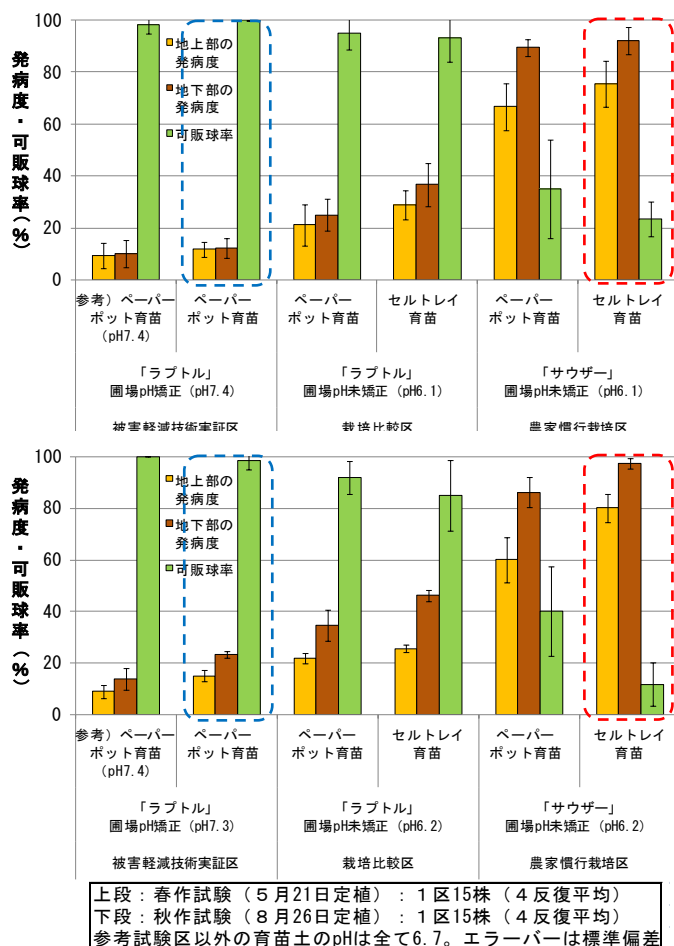
図9. レタス根腐病の被害軽減技術の現地実証結果
